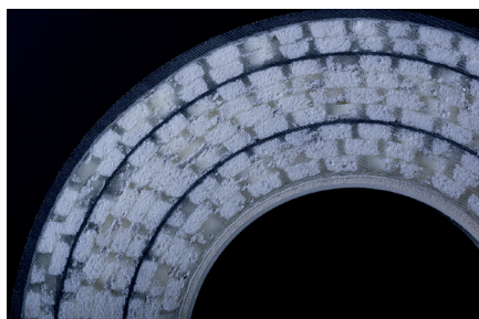
Wabenstrukturaufbau
